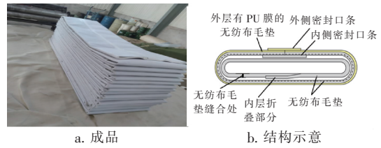
图 3 软管成品及结构示意图
