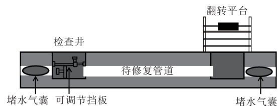
图6 翻转平台的搭建及挡板的安装
