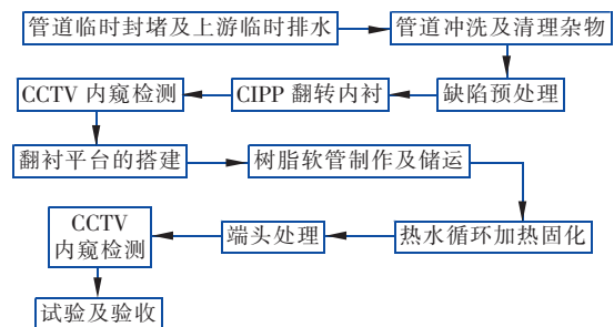
图 4 施工工艺流程
