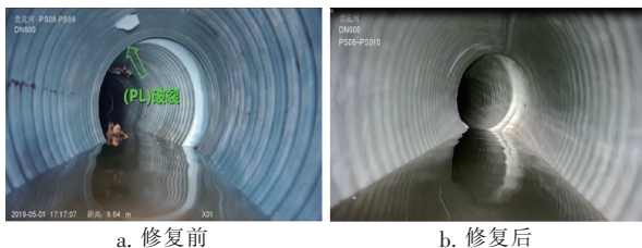
图 7 修复前、后管道内壁形貌
